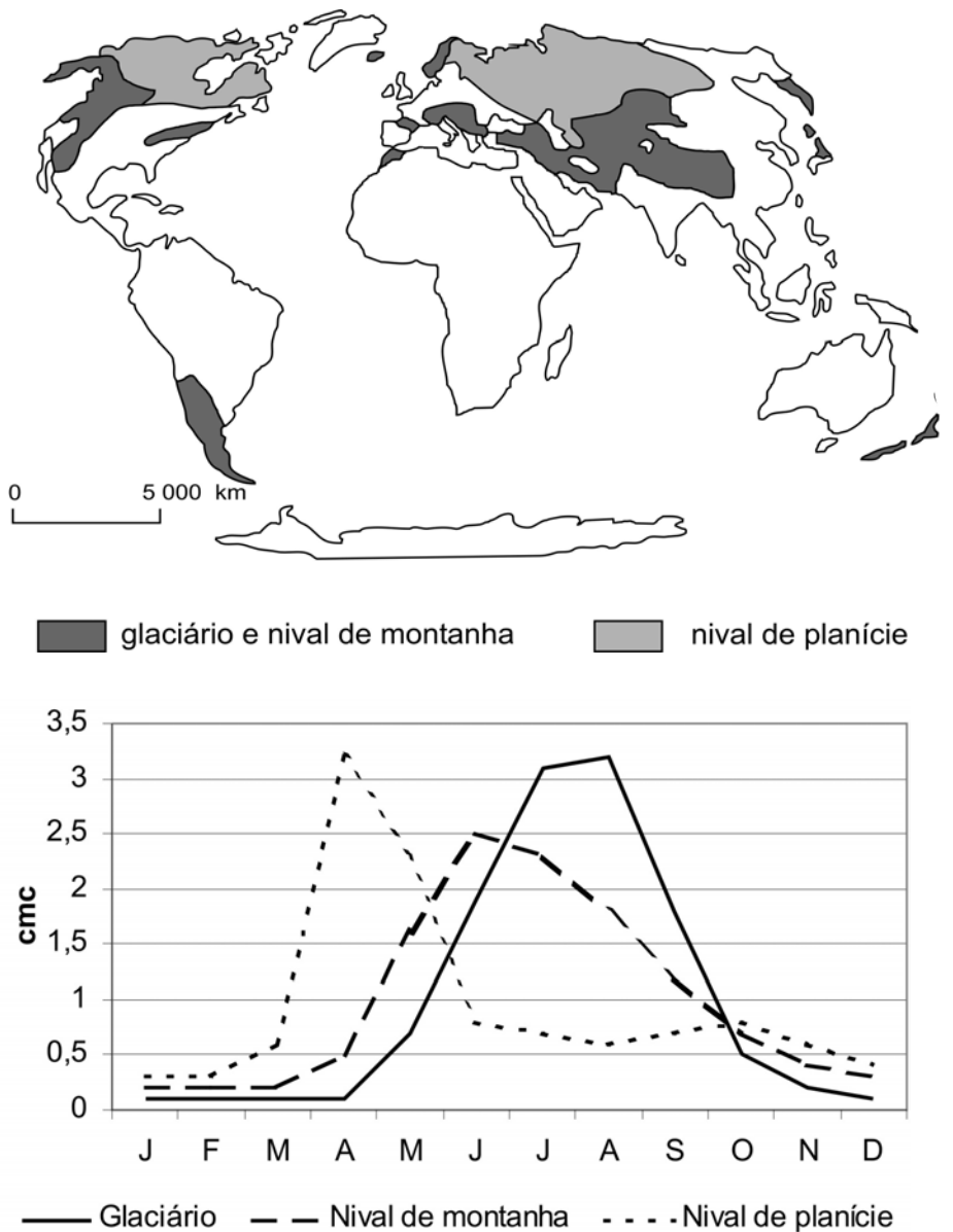
Figura 7 - Os regimes fluviais simples glaciários e nivais: repartição geográfica e variações estacionais.
