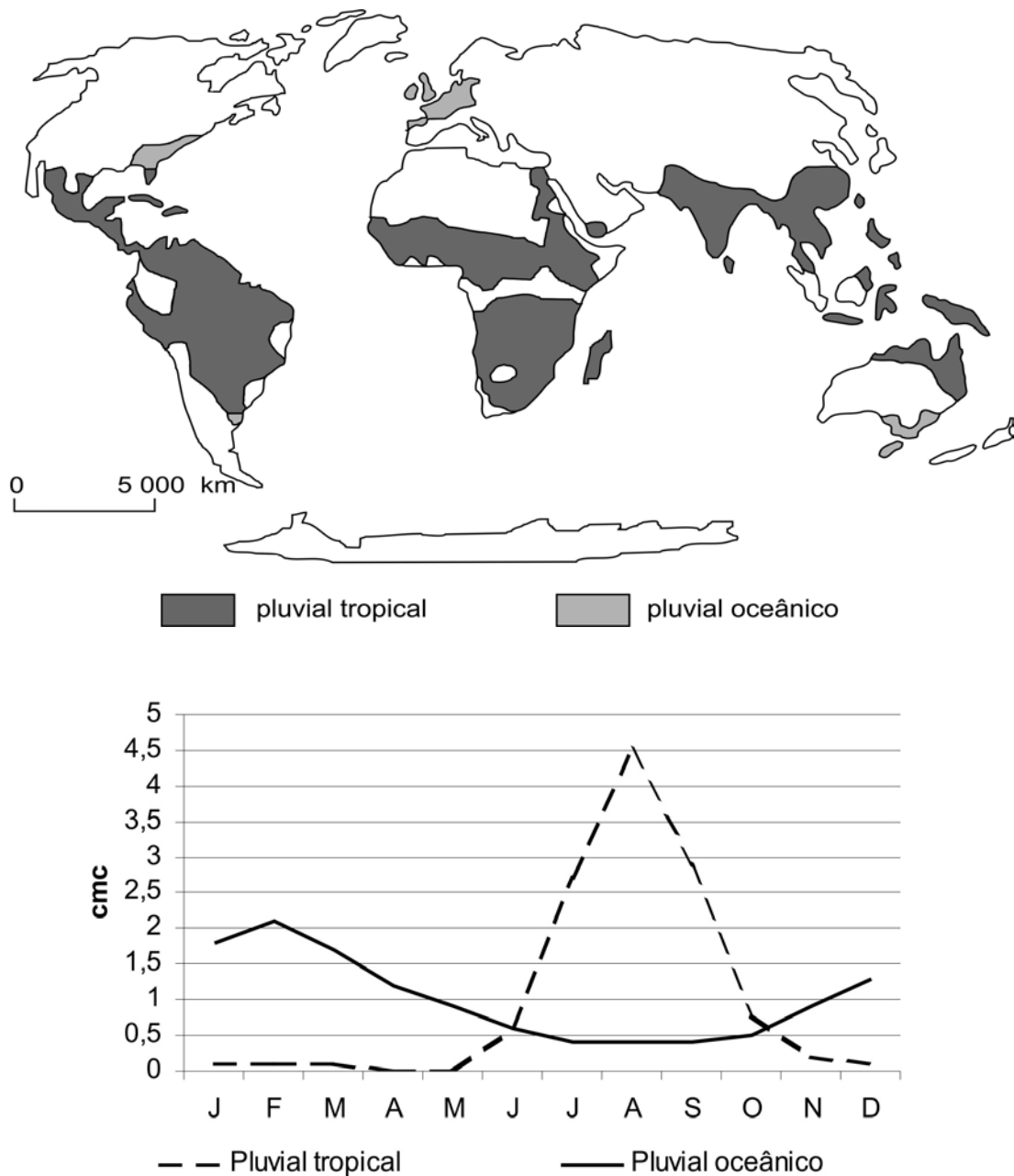
Figura 8 - Os regimes fluviais simples pluviais: repartição geográfica e variações estacionais.
