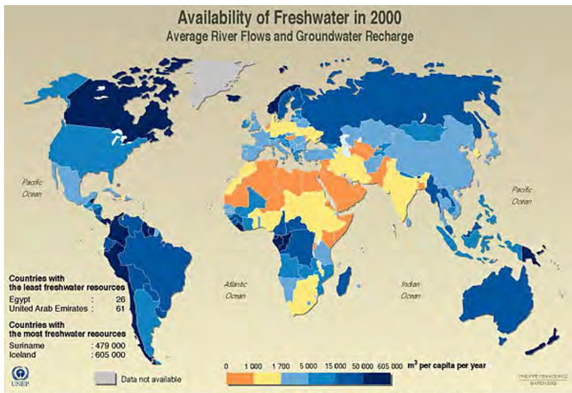
Figura 12 – Disponibilidade de água doce, por habitante / ano, nos diferentes países, no início do século XXI (em: http://freshwater.unep.net/ ).
