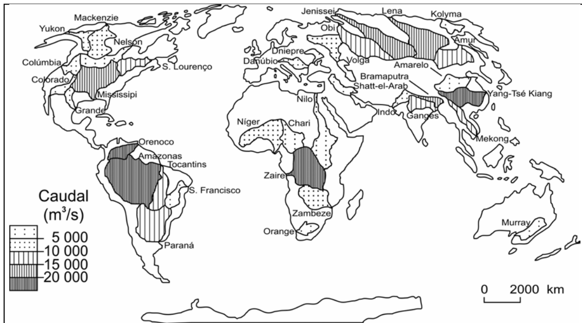
Figura 6 - As grandes bacias hidrográficas do Planeta e caudais anuais (calculados na foz) dos rios que as drenam.
