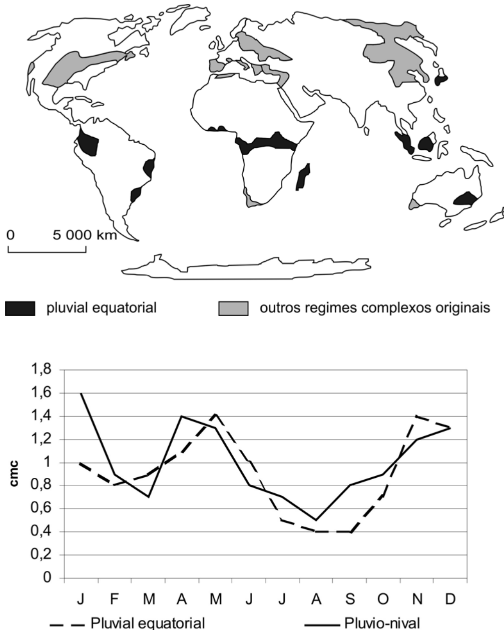
Figura 9 - Os regimes fluviais complexos originais: repartição geográfica e variações estacionais.
