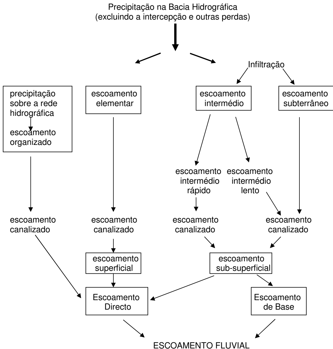
Figura 5 - Diagrama de Ward: as componentes do escoamento fluvial.
