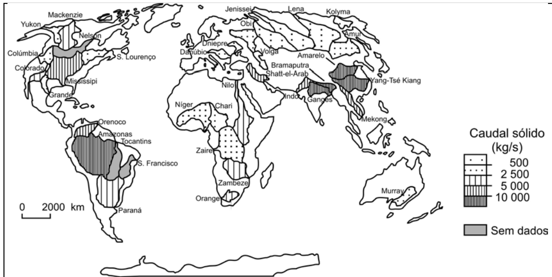
Figura 10 - As grandes bacias hidrográficas do Planeta e caudais sólidos anuais (calculados na foz) dos rios que as drenam.
