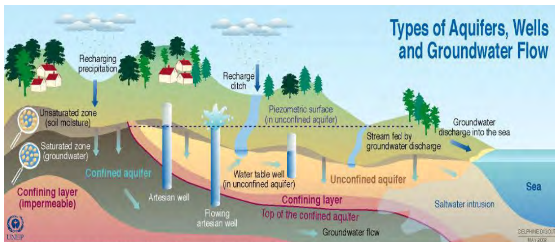
Figura 11 – Tipos de aquíferos (em: http://freshwater.unep.net/ ).
