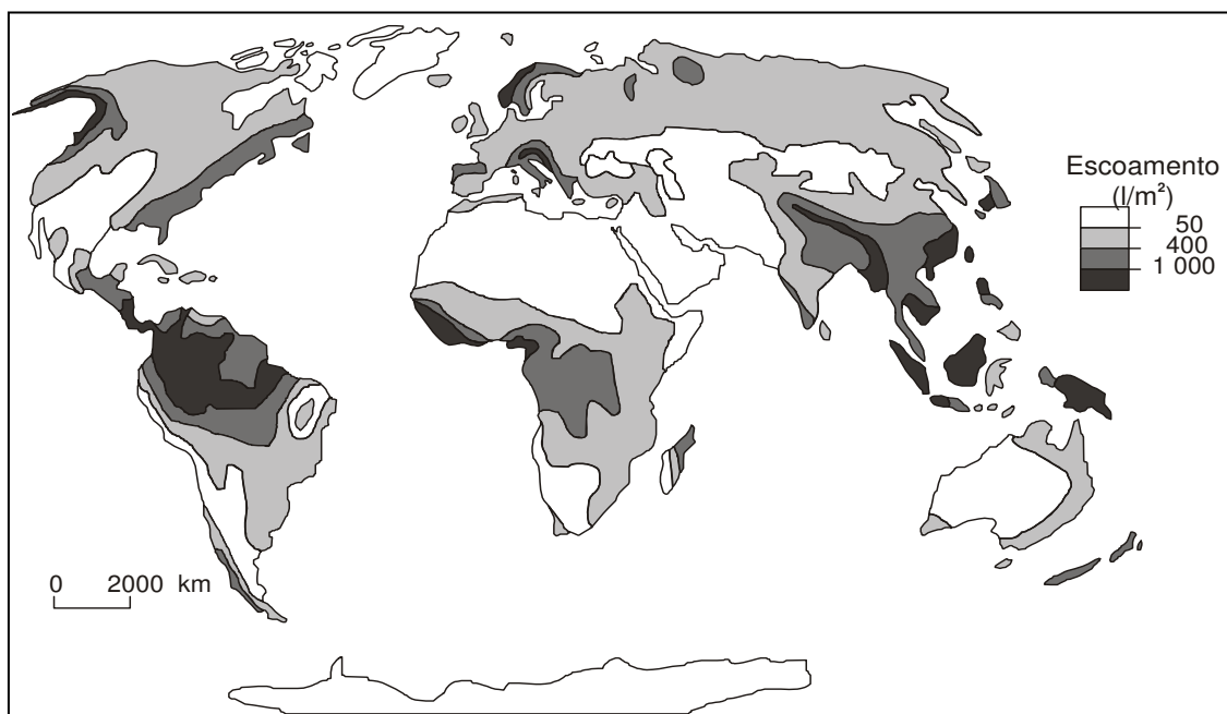
Figura 3 - Repartição espacial do escoamento anual nos diferentes continentes.
