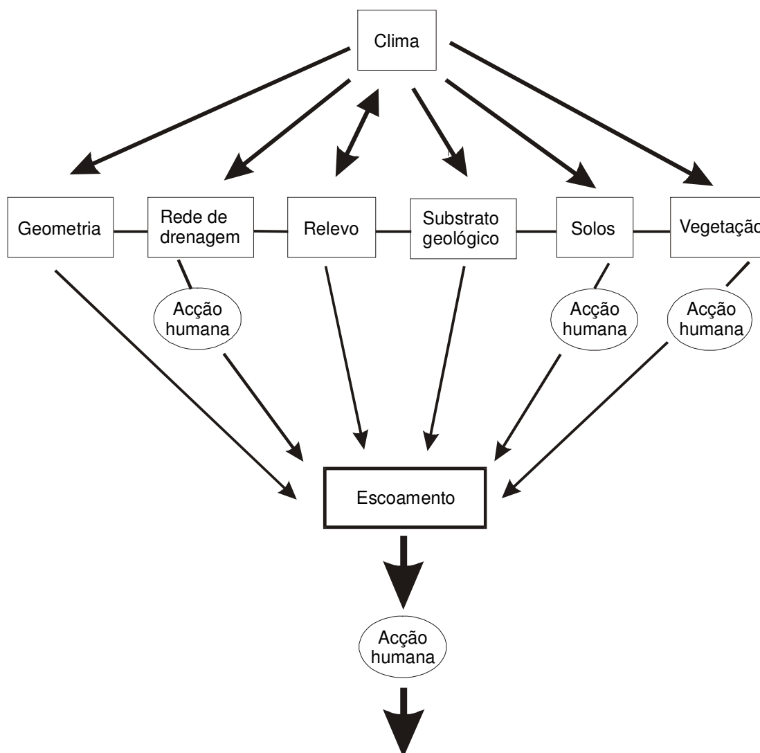
Figura 4 – Factores do escoamento das bacias hidrográficas: enquadramento climático, componentes biofísicas das bacias e intervenção humana.
